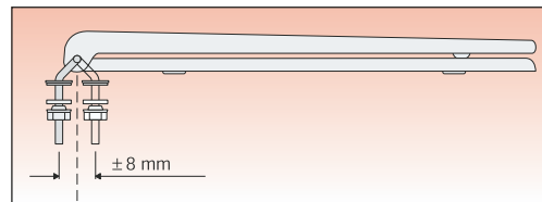
Przekrój deski sedesowej abusanitair wykonanego z Duroplastu
