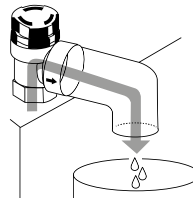
Rys. 1. Montaż zaworu z rurą wyrzutową
