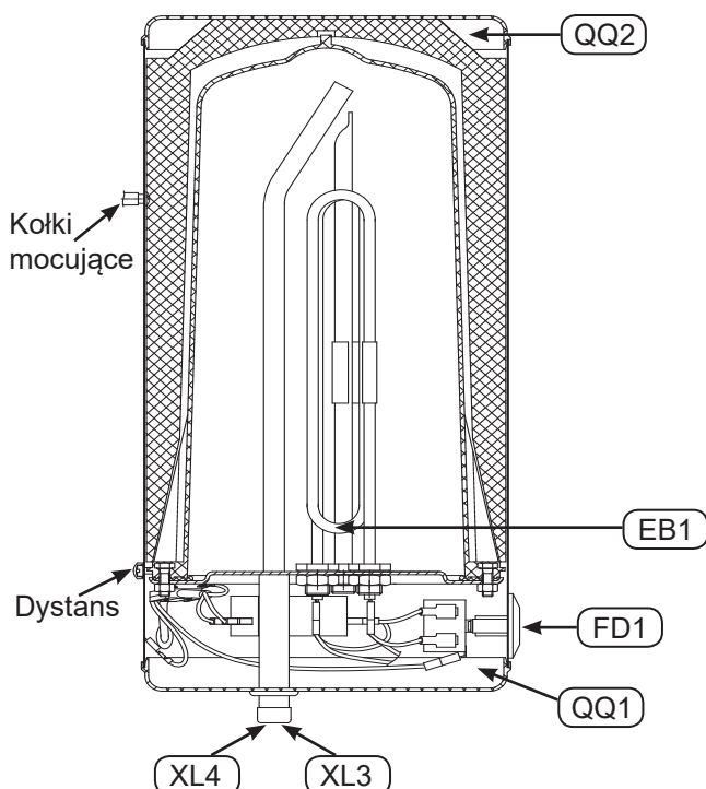
Rys 1. Budowa podgrzewacza
