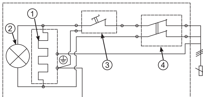
Rys 3. Schemat instalacji elektrycznej podgrzewacza OW-5/10B
