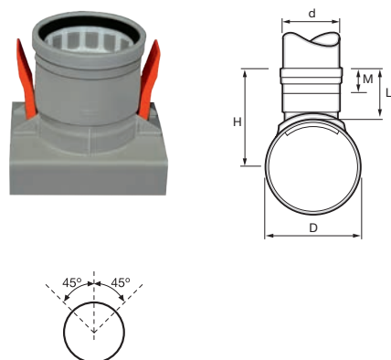
Odgałężenie nasadowe do bezpośredniego włączenia przykanalika do rury gładkościennej - Typ 2 - Kielich Wavin
