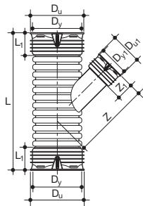
Trójnik redukcyjny 45°
