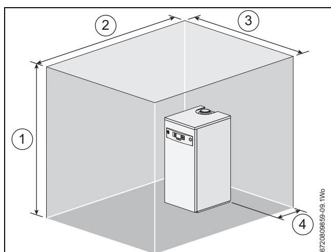
Rys. 13 Odstępy montażowe
