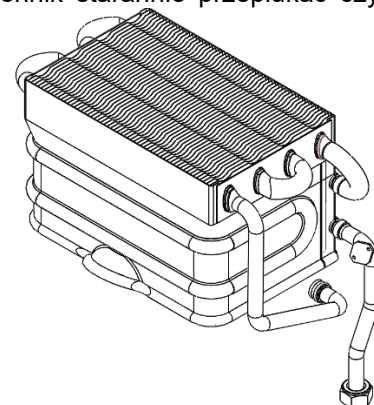
Rys. 6.1.1. Wymiennik ciepła
