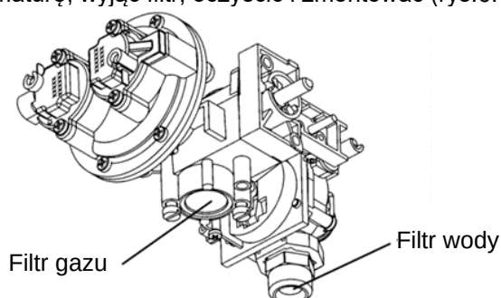
Rys 6.4.1. Armatura wodno-gazowa
