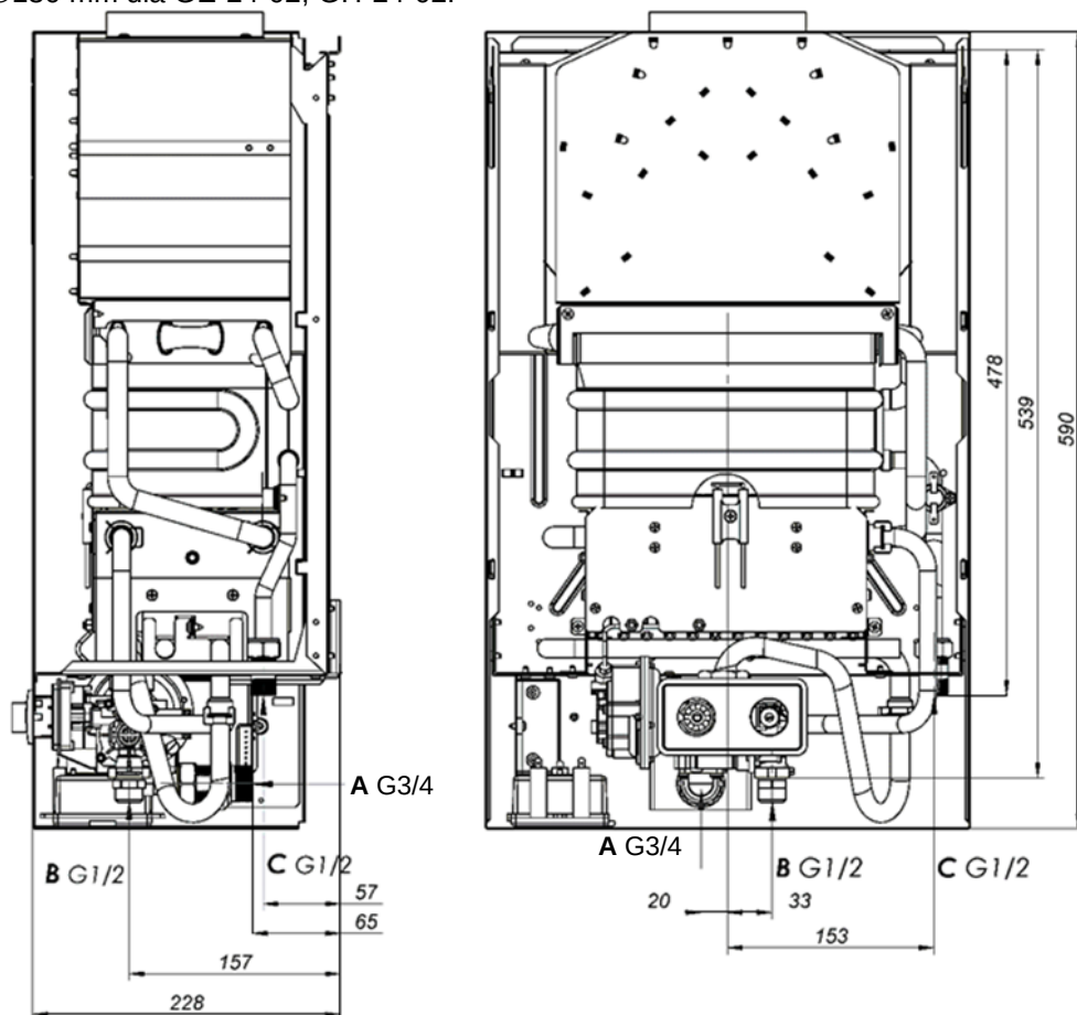
Rys. 3.6.1. Główne wymiary instalacyjne (w mm).
