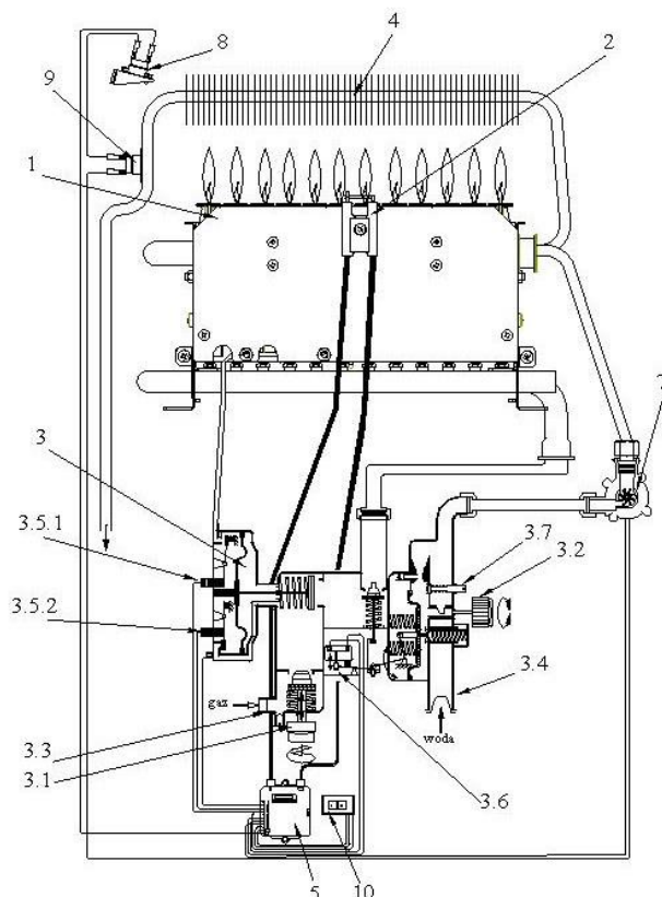
Rys. 2.2.1.2 Schemat ideowy ogrzewacza
